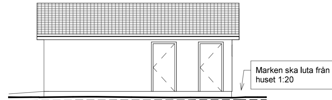
2 Fasad mot öster 1 : 100
