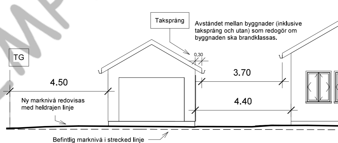
4 Fasad mot söder 1 : 100
