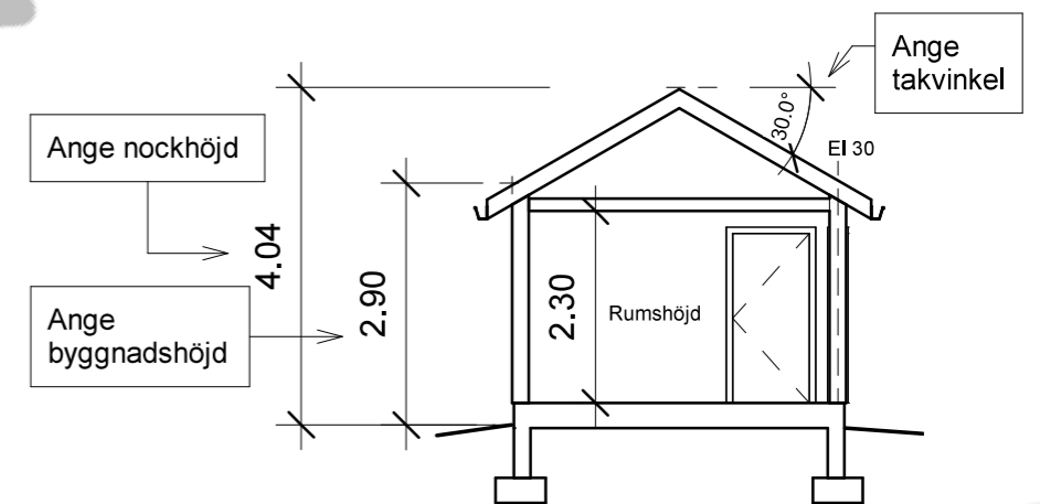
5 Sektion 1 : 100
