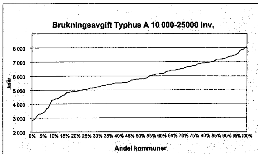
Diagrammet baseras på frågan ba10.
